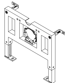
VISTA ISOMÉTRICA
